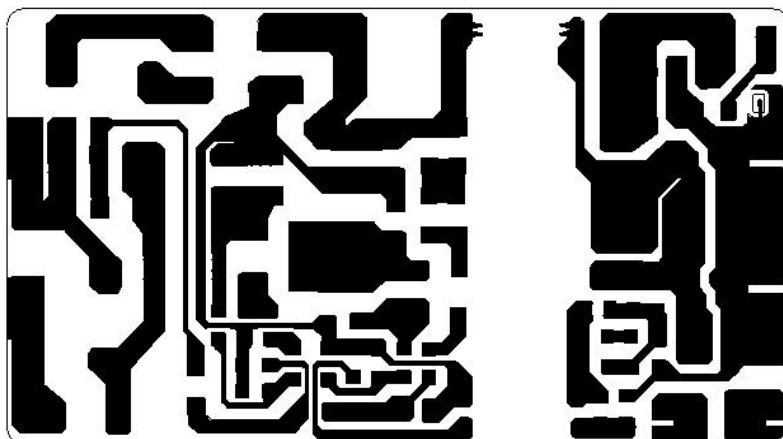
BOTTOM LAYER
