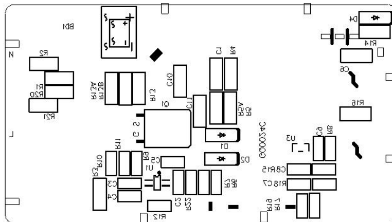
BOTTOM LAYER
