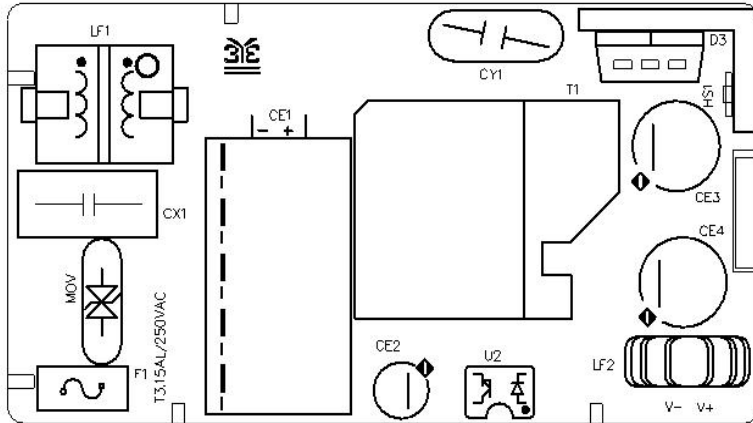
TOP OVERLAY
